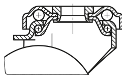
转动环支承：
