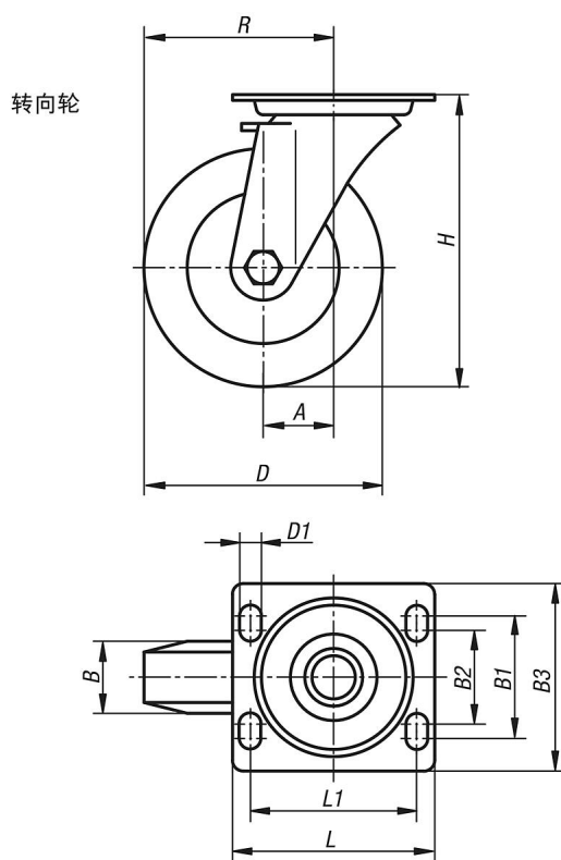
转动环支承：
