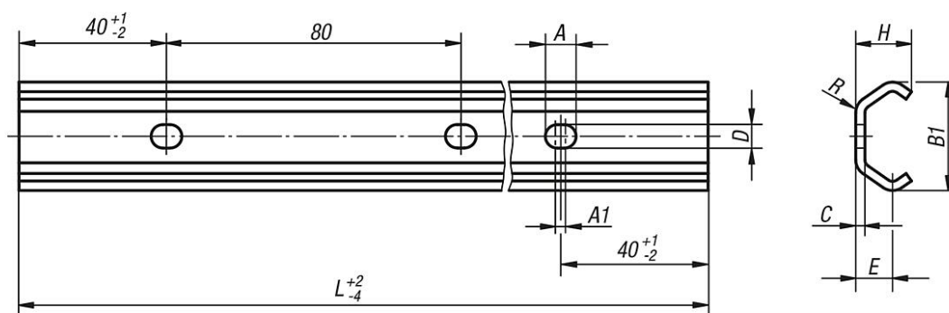
固定滑块的 滚子导轨
