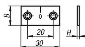
零位标记
