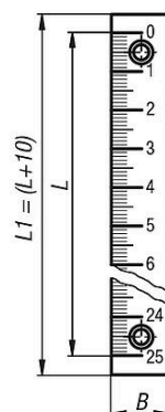
带孔 垂直安装位置
