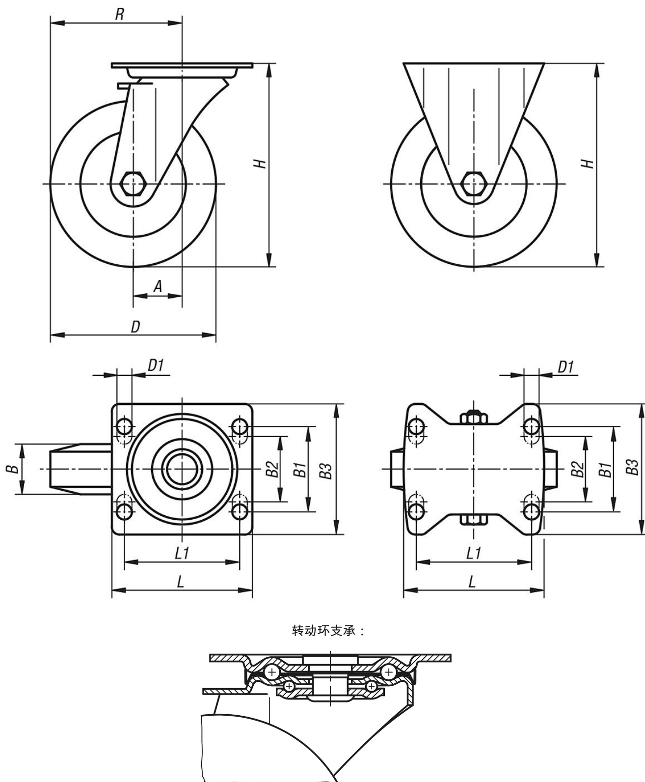
转向轮
