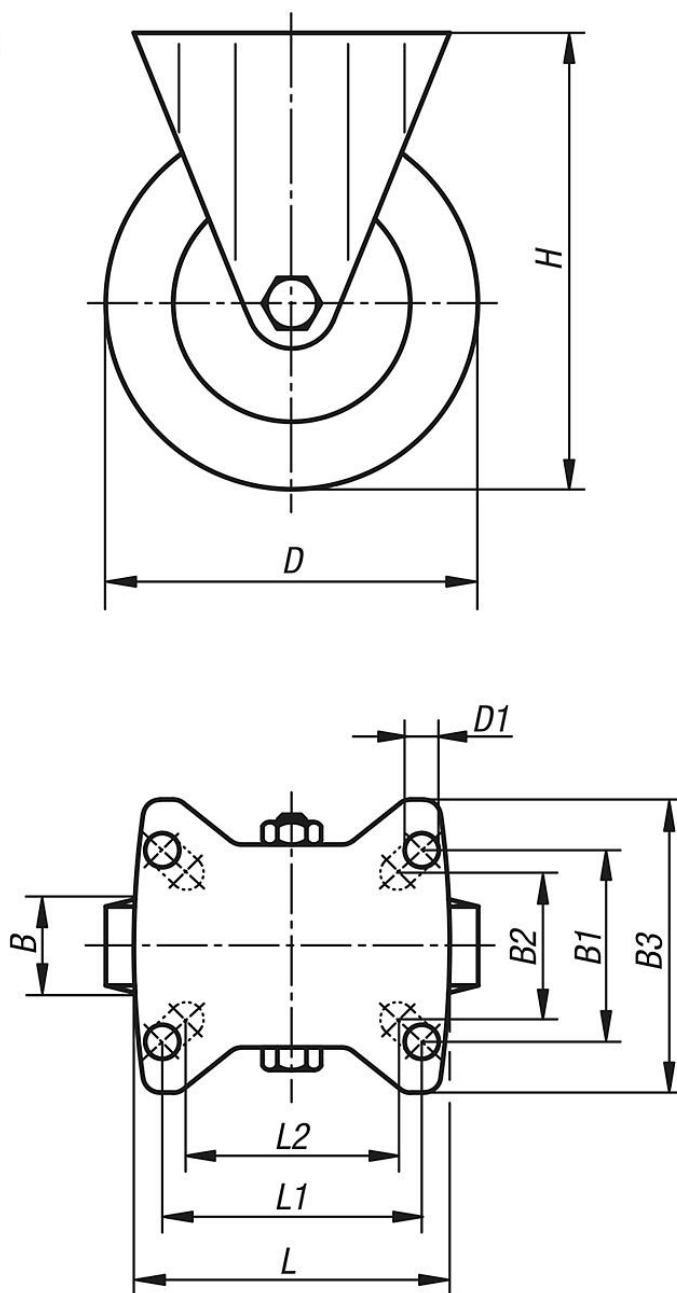
脚轮
