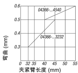
夹紧时 弯曲的夹紧臂长度 C
