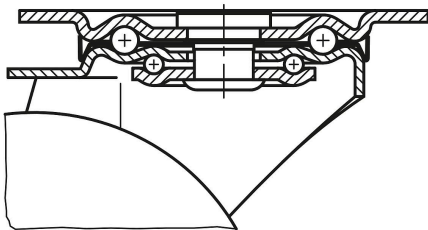
转动环支承：
