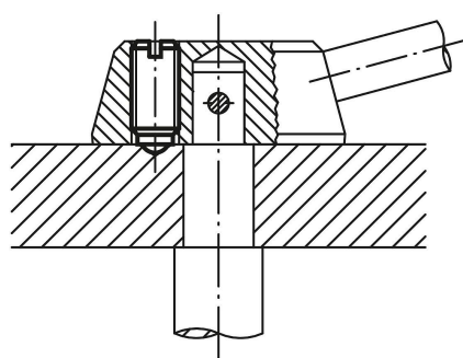
把手分度
