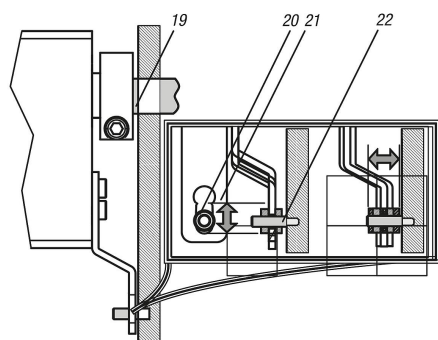
装配:
